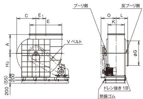
TV-L 型
