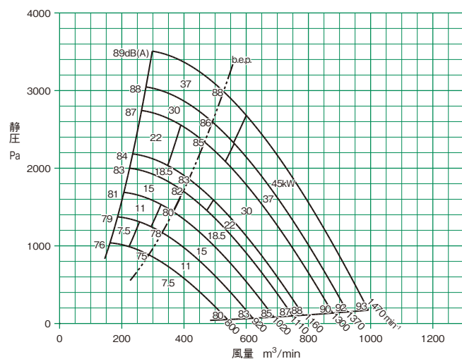
ETF(R)-No.7b
