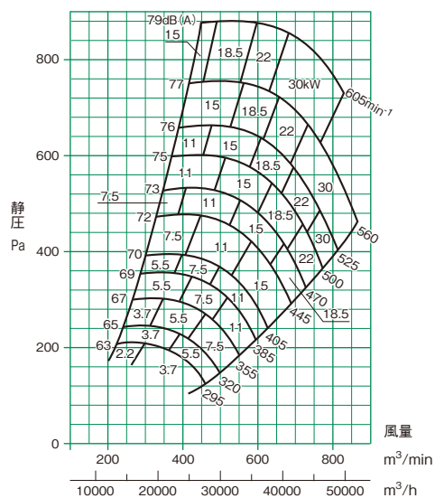
No.5½
