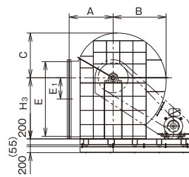
BH-L 型
