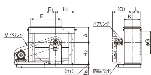
TV-R 型
