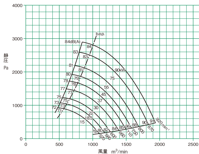
ETF(R)-No.9
