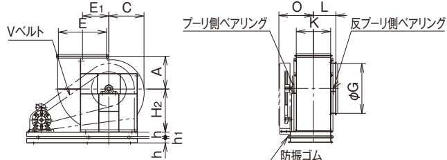
TV-L 型
