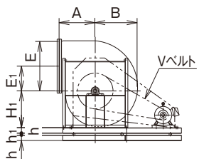
TH-L 型
