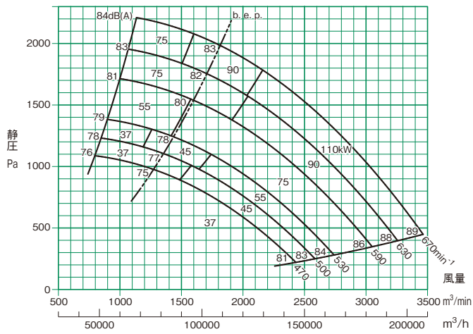
CMF3(R)-No.11
