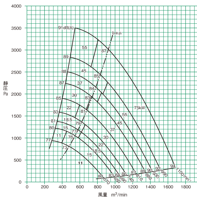
ETF(R)-No.8
