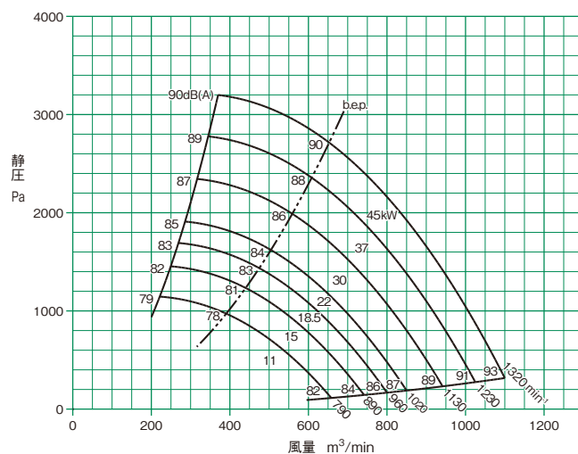
ETF(R)-No.8
