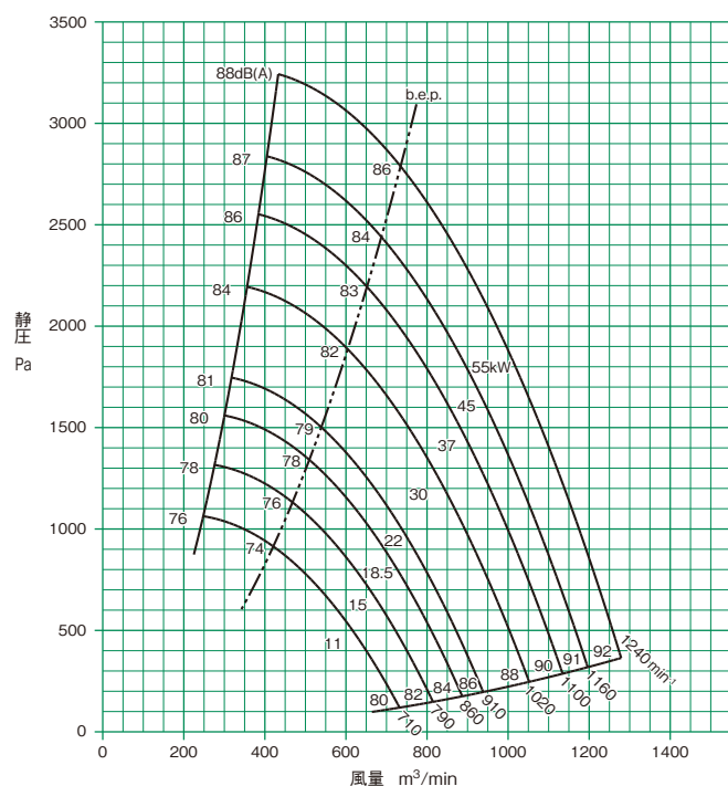
ETF(R)-No.9
