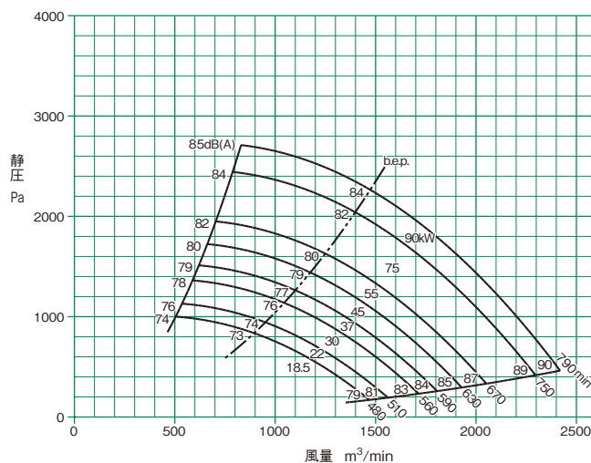
ETF(R)-No.10
