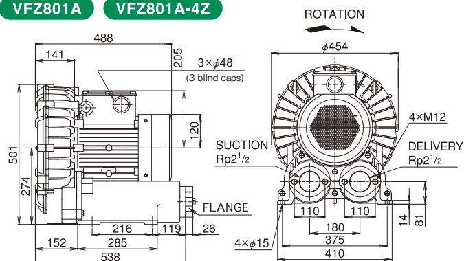
VFZ801A
