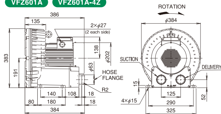
VFZ601A
