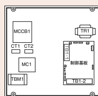
制御盤の機器構成(直入起動BN3L)
