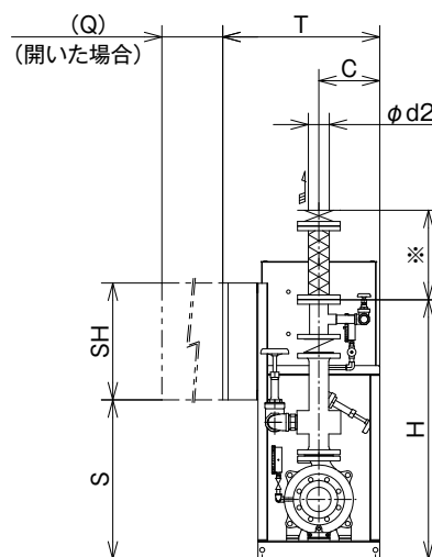
X-X矢視図
