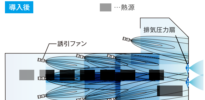
場内換気促進用 誘引ファン
